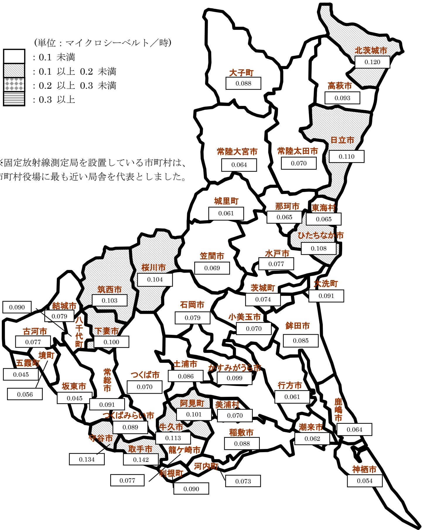
第21回 (H24. 3. 14) 全市町村放射線量率測定結果
