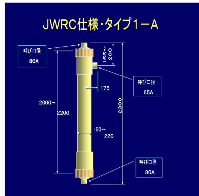
膜モジュールJWRC仕様の例
