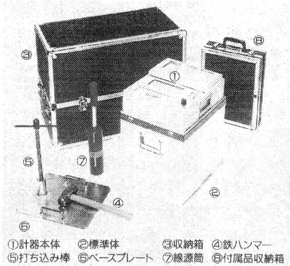
図-4 計器の構成例（透過型）
