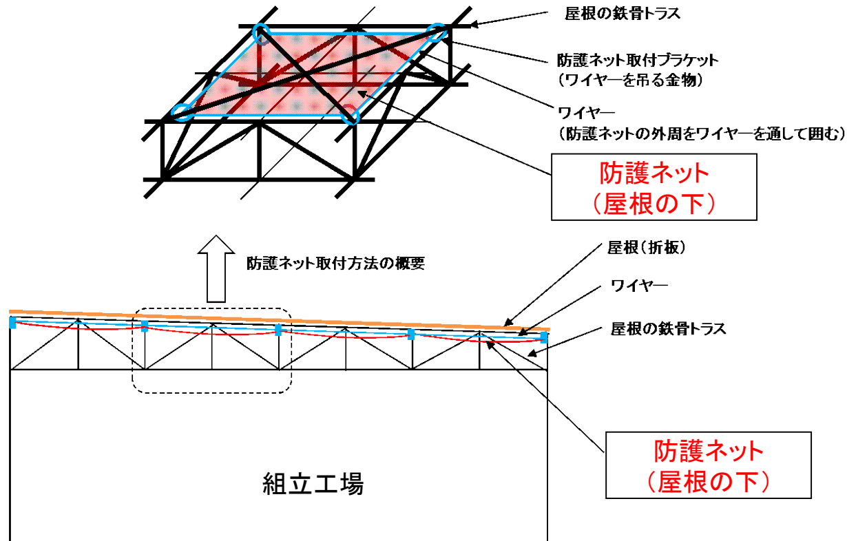
気圧差による影響対策(例)
