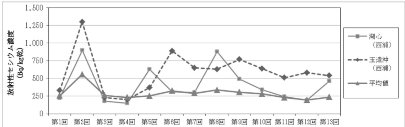
第13回調査において放射性セシウム濃度の高い地点の数値の推移 (セシウム134+セシウム137)
