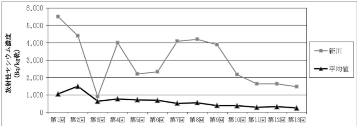
第13回調査において放射性セシウム濃度の高い地点の数値の推移 (セシウム134+セシウム137)
