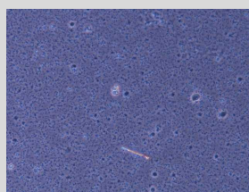
図2. PCM法での観察画像
