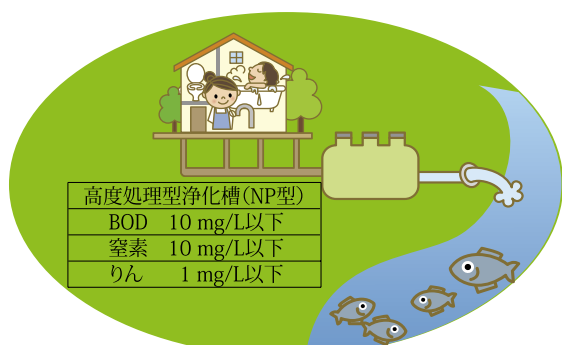
通常型浄化槽と高度処理型浄化槽の放流水比較図
