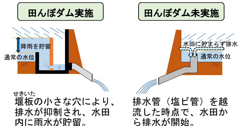
田んぼダム用の落水柵
