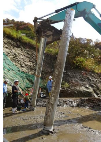
支柱引抜試験
