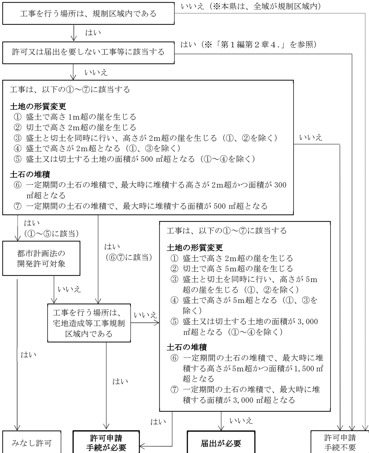
図 1.6 盛土規制法に基づく許可要否の判定フロー
