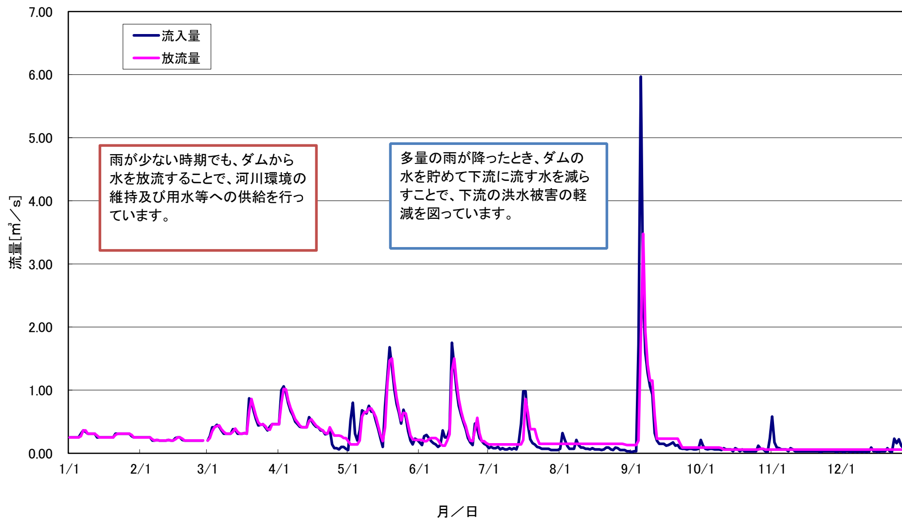
令和7年 飯田ダムの流入量・放流量(日平均)
