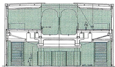
■駅舎断面図
