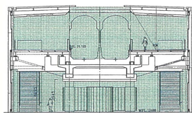
■駅舎断面図
