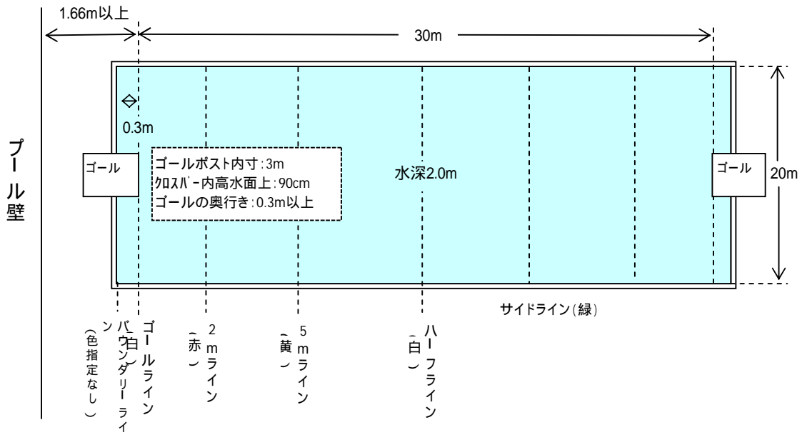
【別図2】水球用プール
