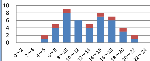
国道355号における時間別・危険認知速度別人身交通事故の発生状況(過去3年間)
