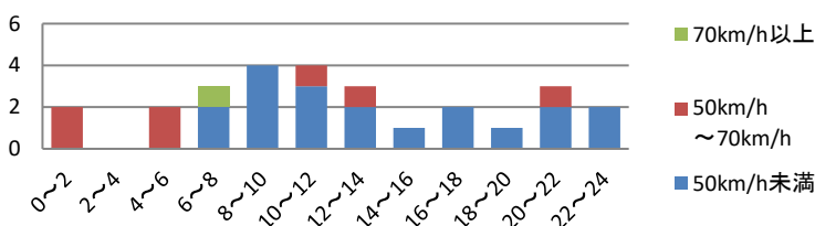
国道294号における時間帯・危険認知速度別 事故の発生状況(過去3年間)
