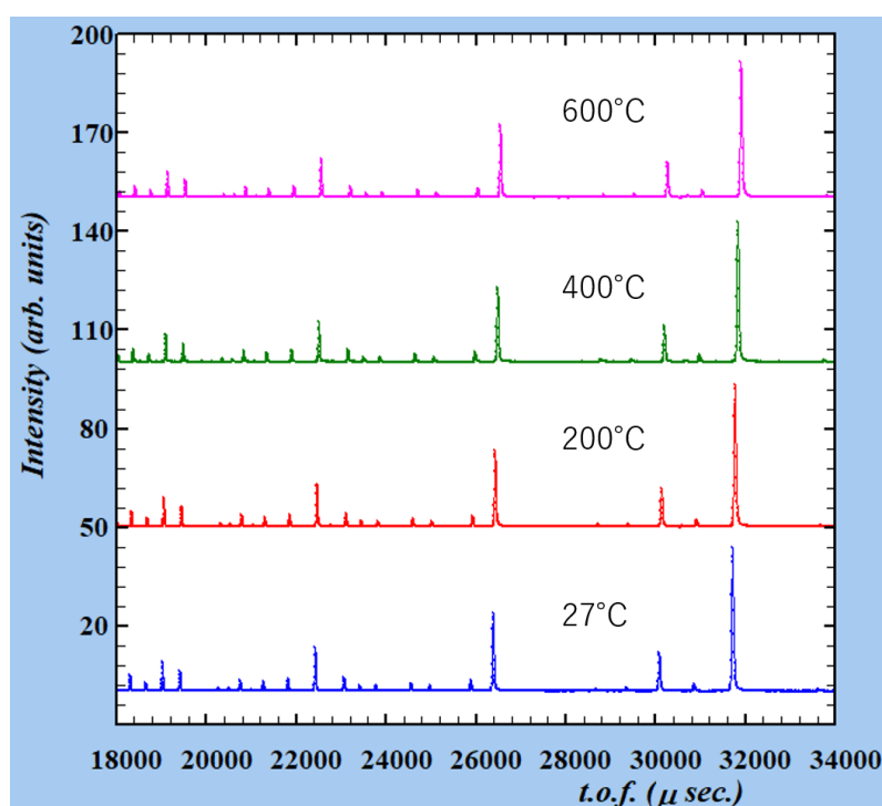
図1：あるイオン伝導体の室温から高温にかけて測定した回折パターン。
