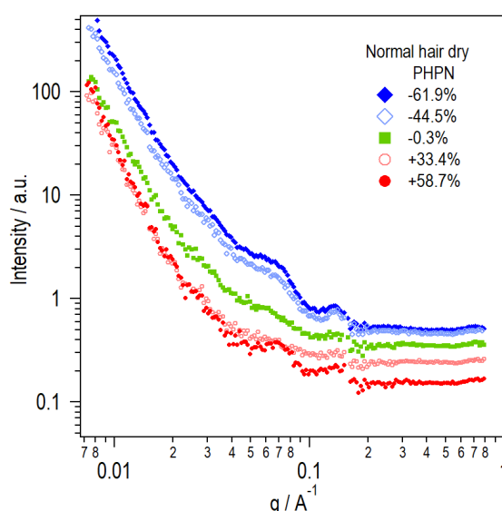
図2. 乾燥毛髪の中性子小角散乱プロファイル。核スピン偏極の適用によりコントラストを制御している
