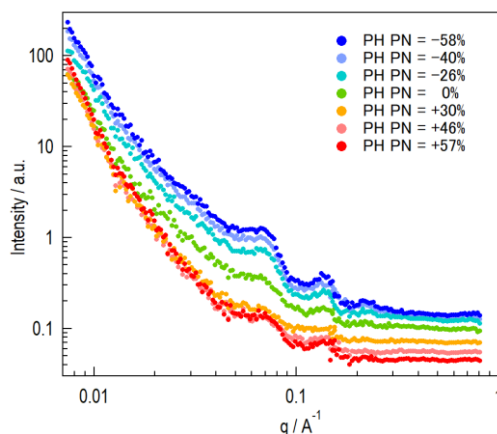
図2. 白髪の中性子小角散乱プロファイル。核スピン偏極の適用によりコントラストを制御。
