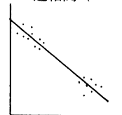
逆相関 ( r < 0 )
