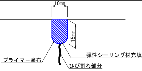
標準断面図 (ひび割れ充填工法)
