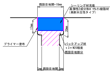
標準断面図 (目地充填工法)
