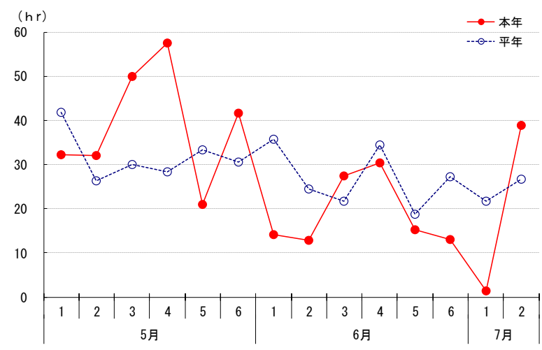
図2 半旬別日照時間の推移（土浦市） 注）平年値：平成28年～令和7年の10年間の平均値 アメダス土浦龍観測所データより作成
