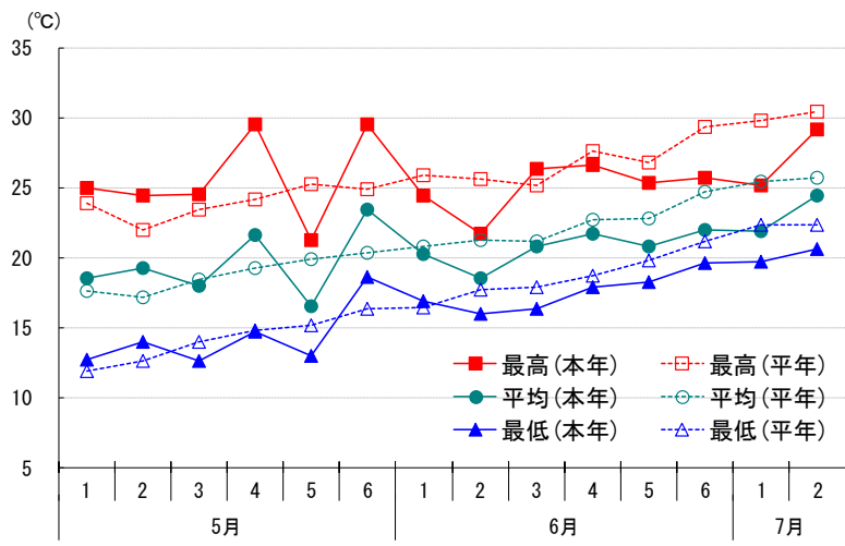
図1 半旬別気温の推移（土浦市） 注）平年値：平成28年～令和7年の10年間の平均値 アメダス土浦観測所データより作成
