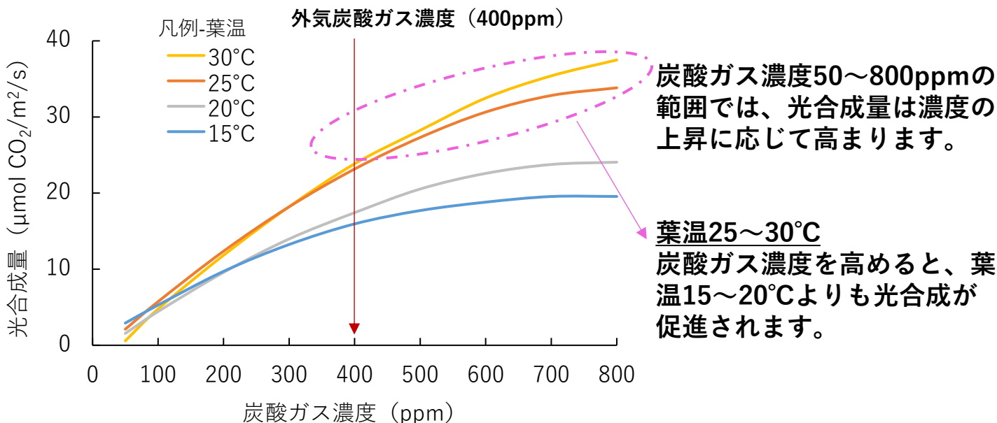
図2 晴天時 (日射量 720\text{W}/\text{m}^2 ) における葉温と炭酸ガス-光合成曲線の関係 (2021年、鹿島特産)
