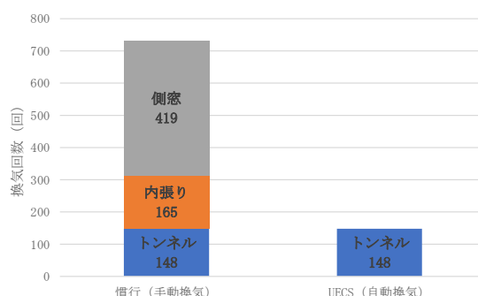
メロン1作中の換気回数の比較※（手動換気ハウス（左）、UECSを活用した自動換気ハウス（右））※ハウス1棟あたり
