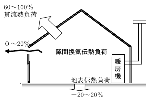
図II-2-1 温室の熱損失
