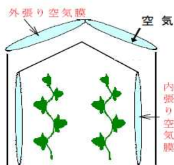
図Ⅱ-2-12 空気膜ハウスの断面図および外観
