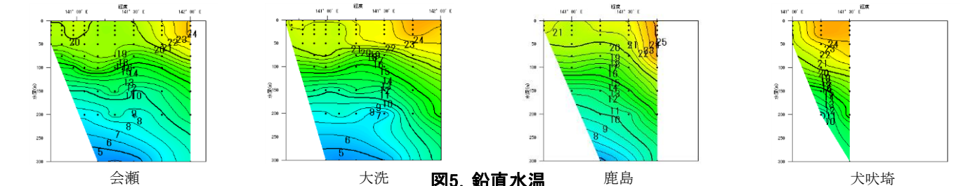
図5. 鉛直水温
