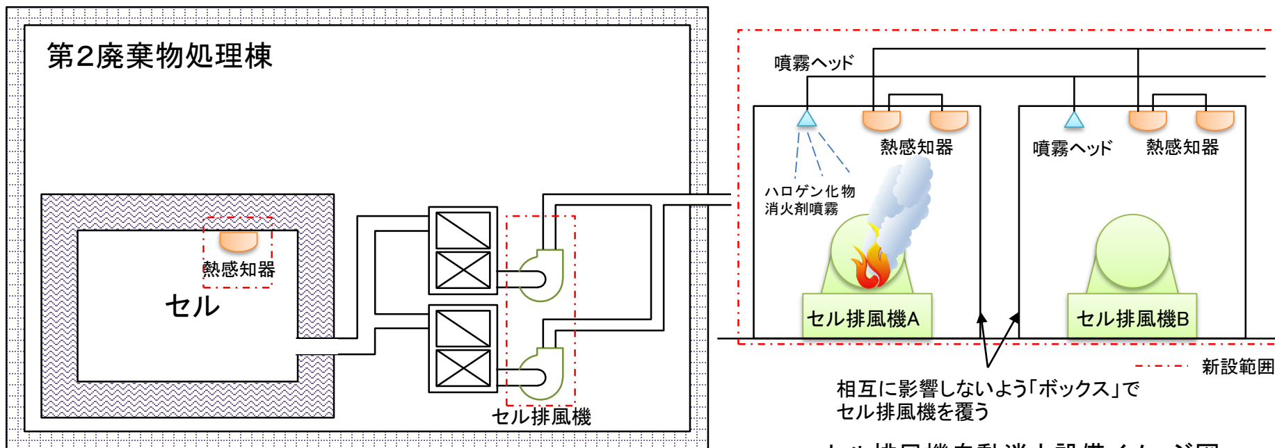
セル排風機自動消火設備イメージ図
