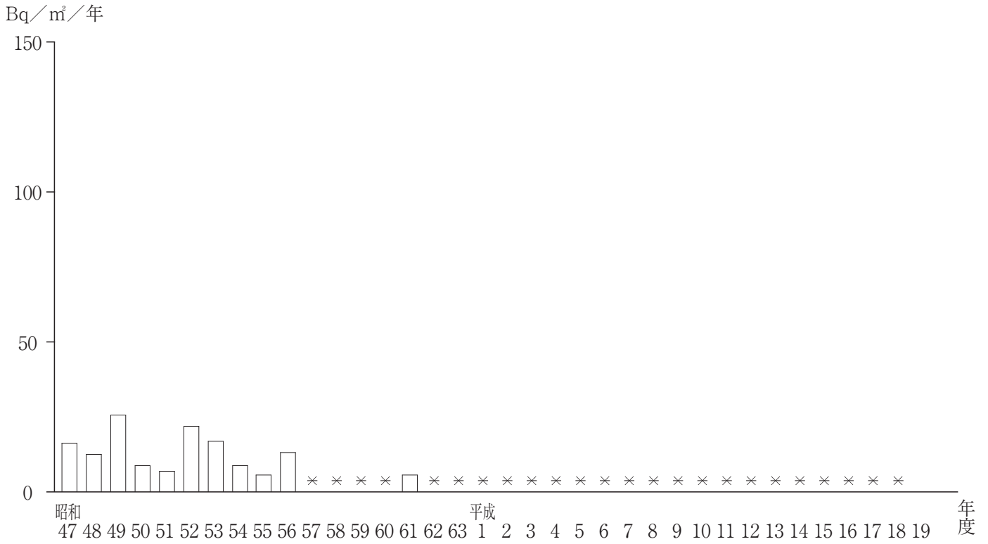
降下塵中のSr-90経年変化【水戸】
