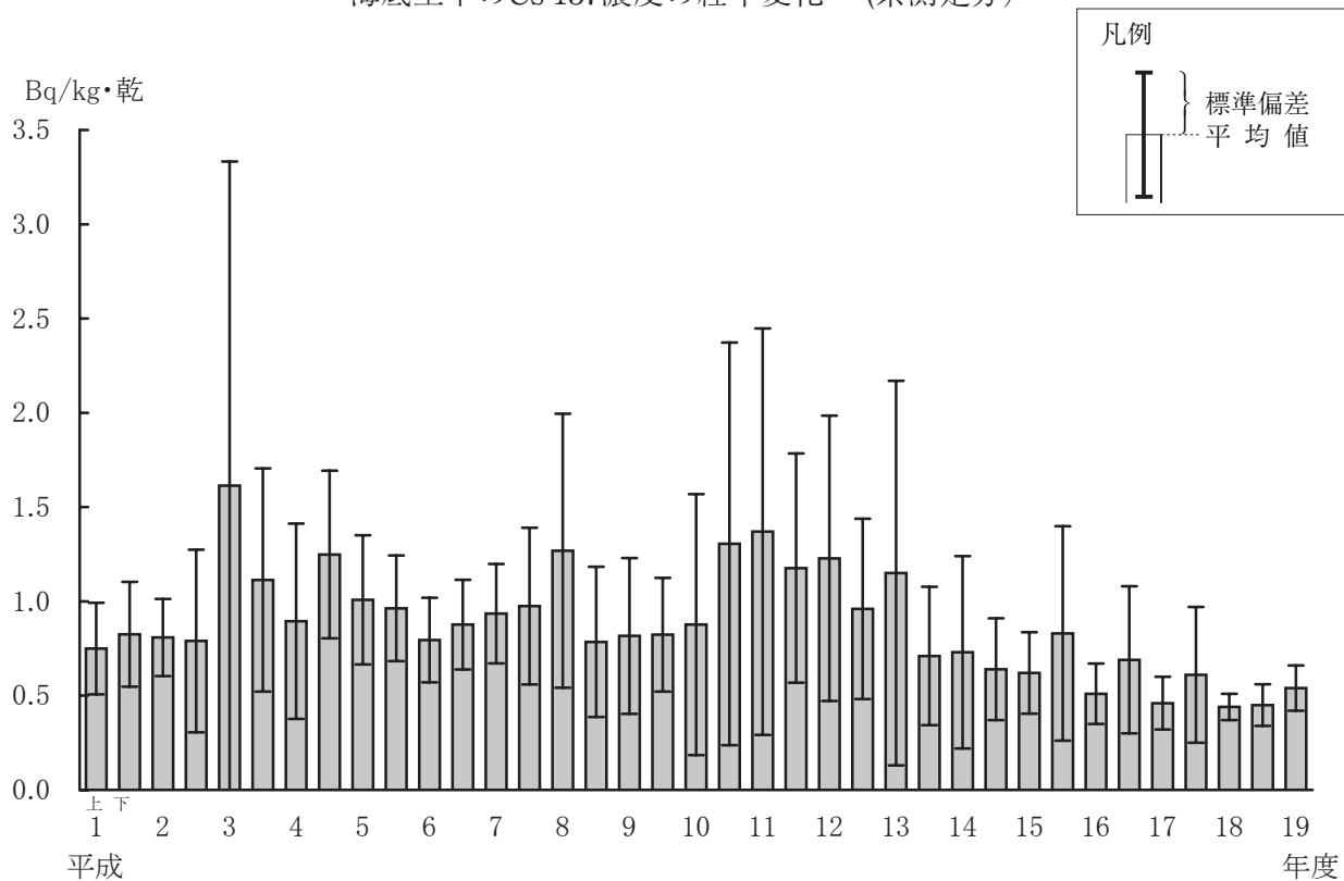
海底土中のCs-137濃度の経年変化 (県測定分)
