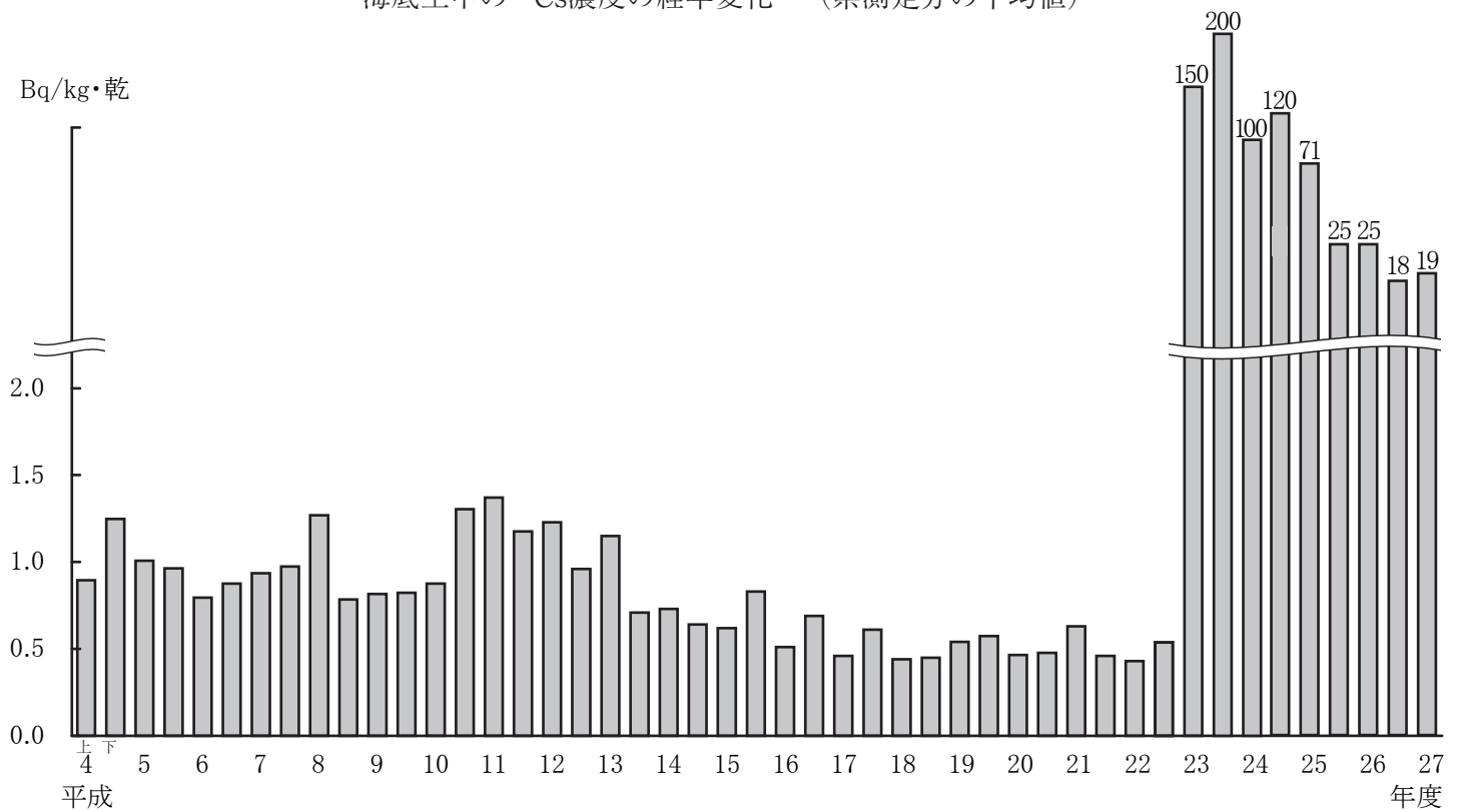
海底土中の 137 Cs濃度の経年変化 (県測定分の平均値)
