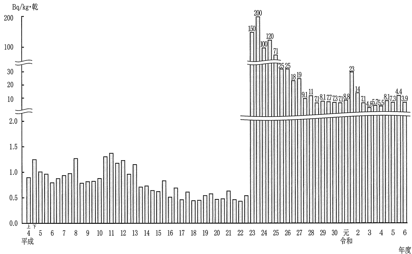
海底土中の ^{137}\text{Cs} 濃度の経年変化 (県測定分の平均値)
