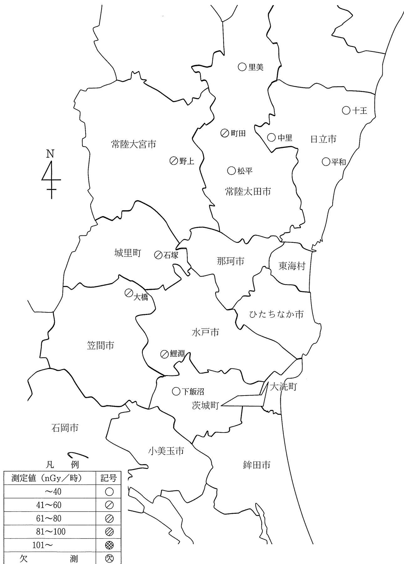
図2 原電から10~30km圏内地区における空間 \gamma 線量率測定結果(3か月平均値)
