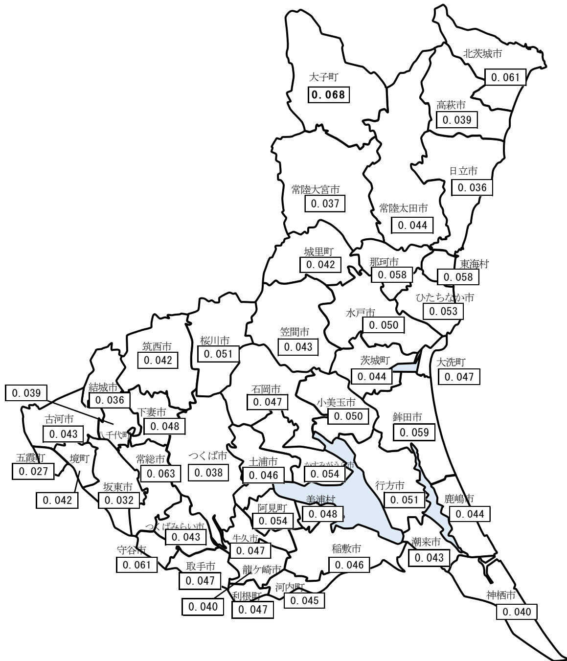
図Ⅱ-1 令和7年12月31日12時における全市町村放射線量率測定結果（地上1m） （令和7年12月31日に欠測となっている局は、直近の測定値を記載）
