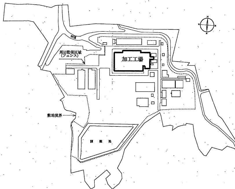
原子燃料株式会社東海事業所 敷地内施設配置置図
