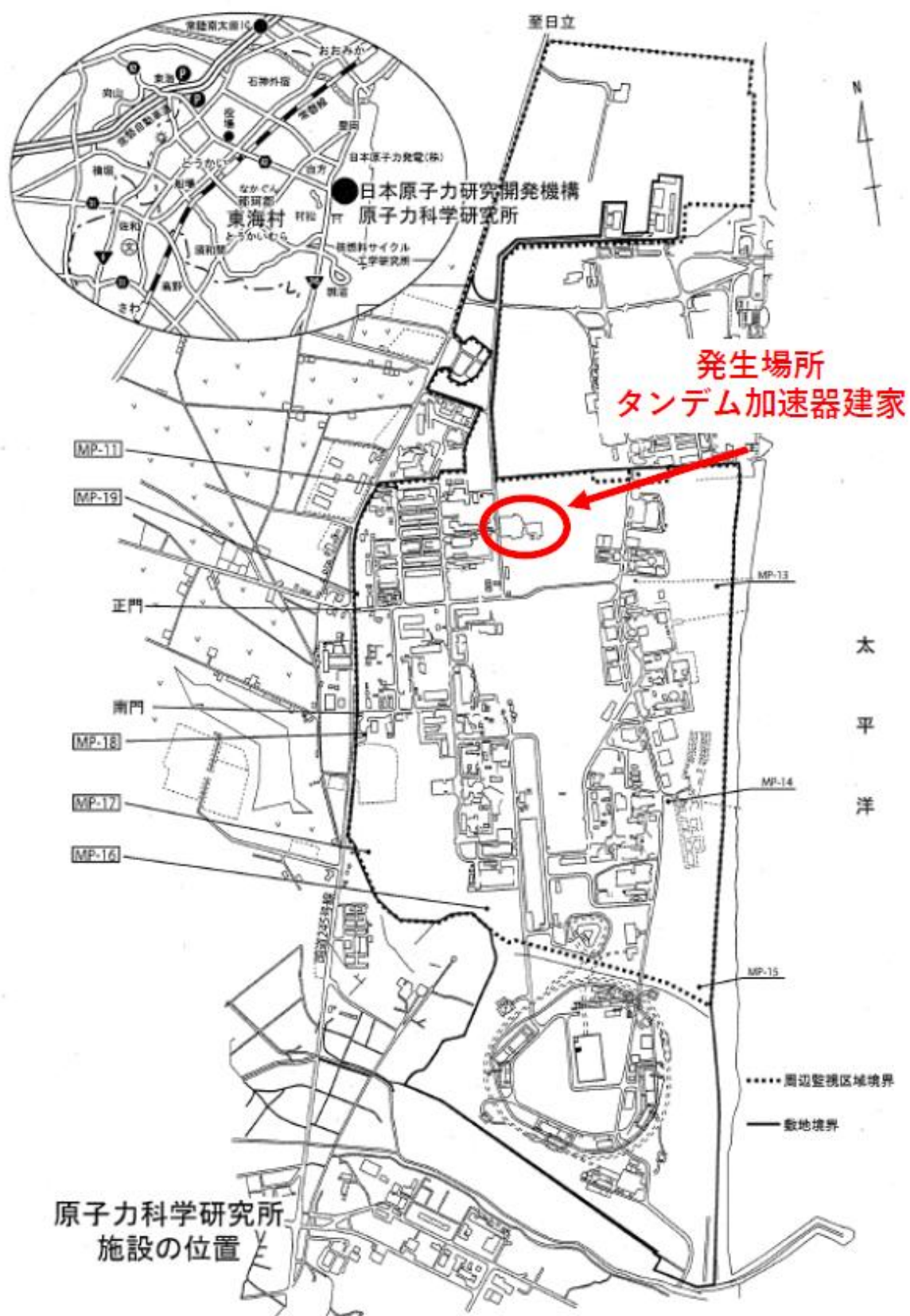
原子力科学研究所 施設配置図
