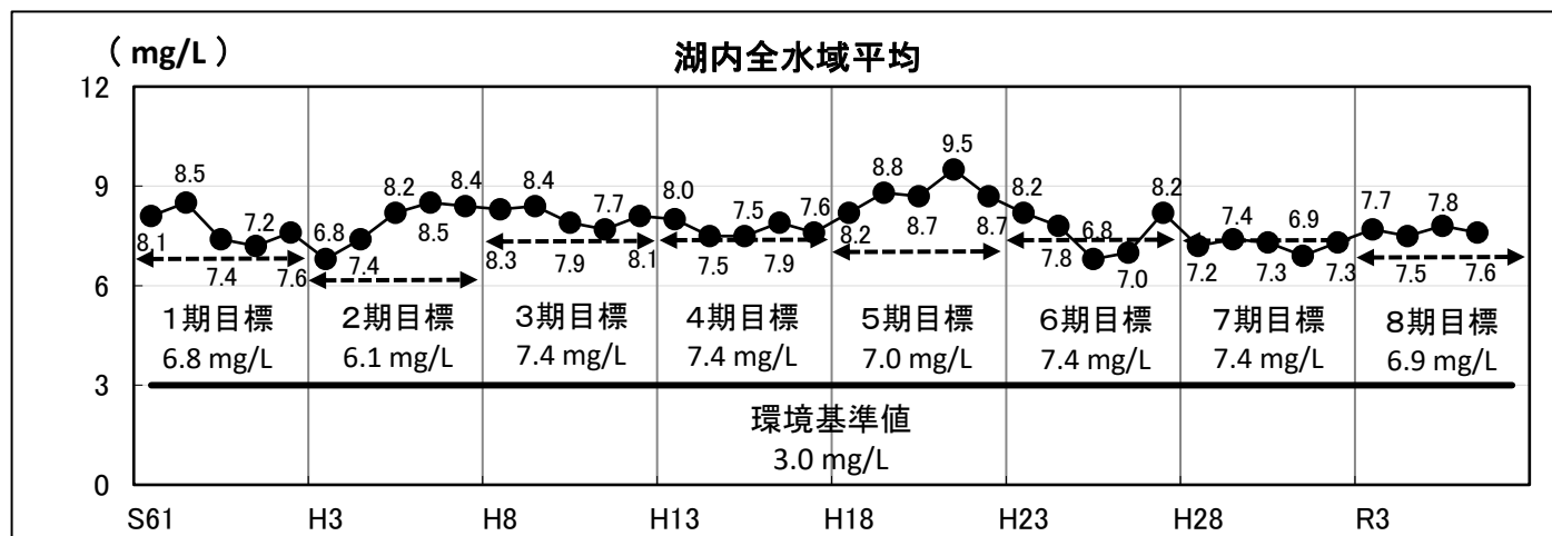
図1 COD(湖内全水域平均)
