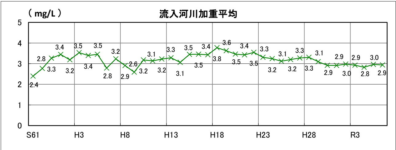
図5 全窒素(流入河川加重平均)
