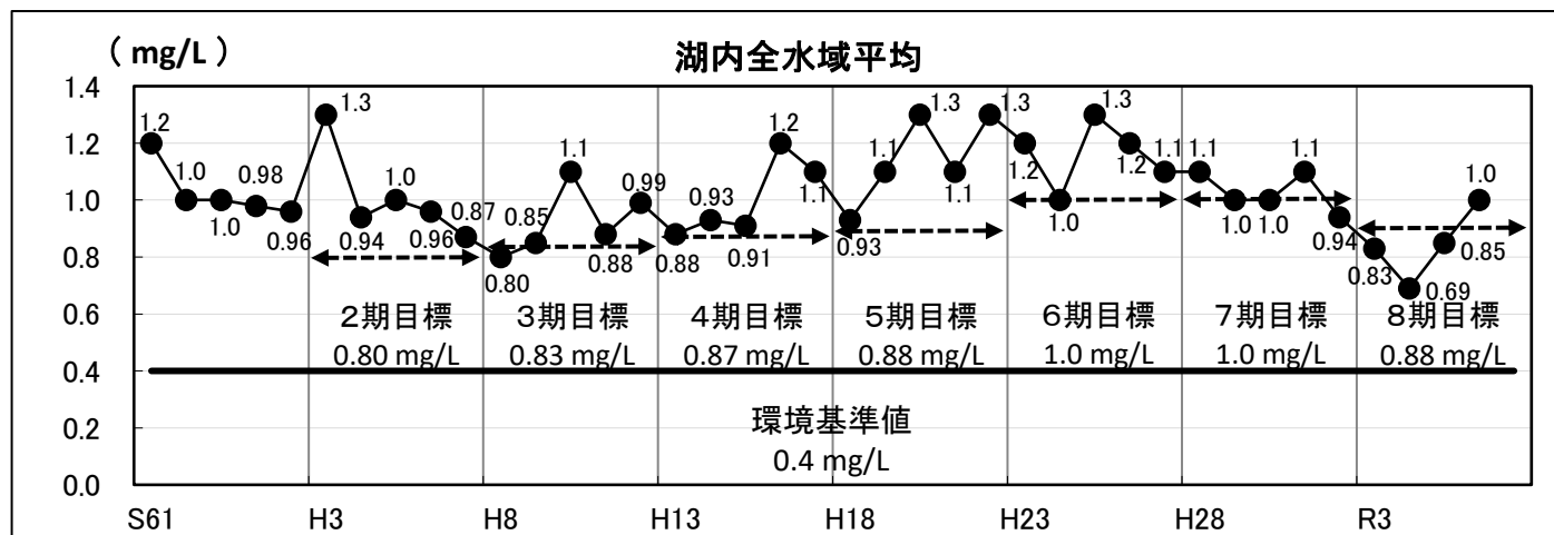
図2 全窒素(湖内全水域平均)
