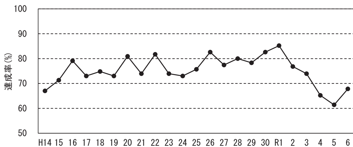
図2 全水域（河川（BOD）及び湖沼・海域（COD））の環境基準達成率の推移
