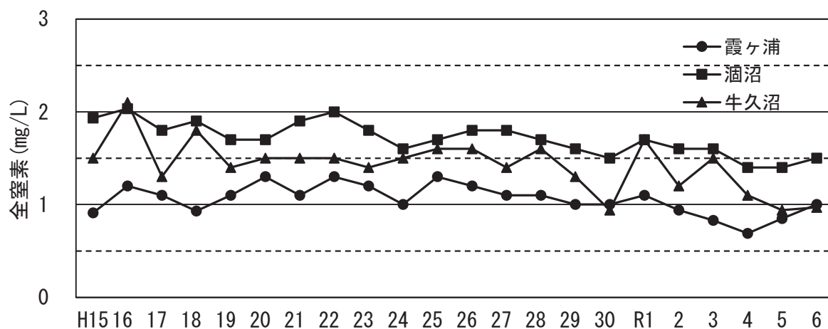
図4 霞ヶ浦、瀬沼及び牛久沼における全窒素（年平均値）の推移
