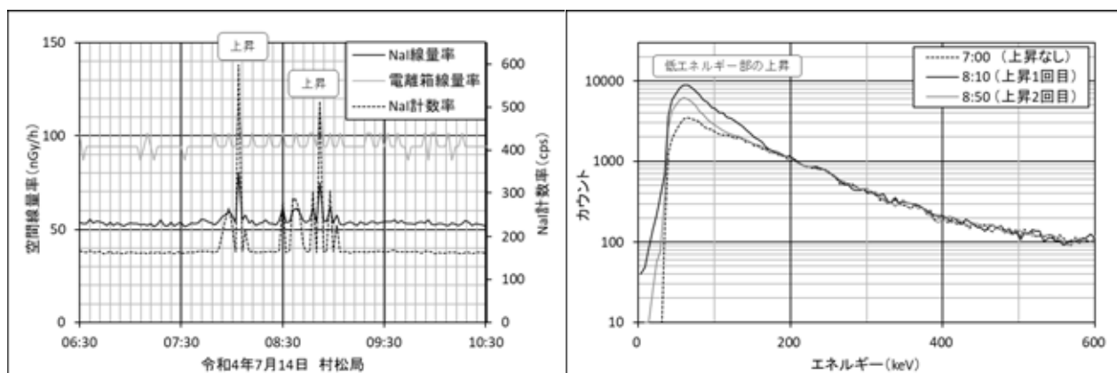
図2 X線非破壊検査による空間線量率 (2分値) の上昇例 左:トレンドグラフ 右:MCA スペクトルグラフ (村松局:令和4年7月14日)
