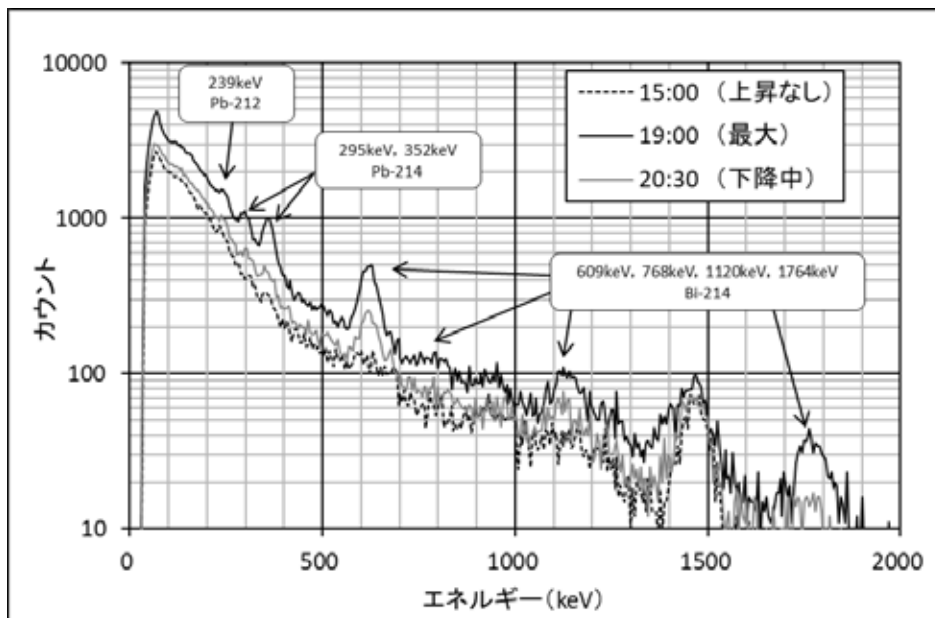
図4 舟石川局のMCAスペクトルグラフ
