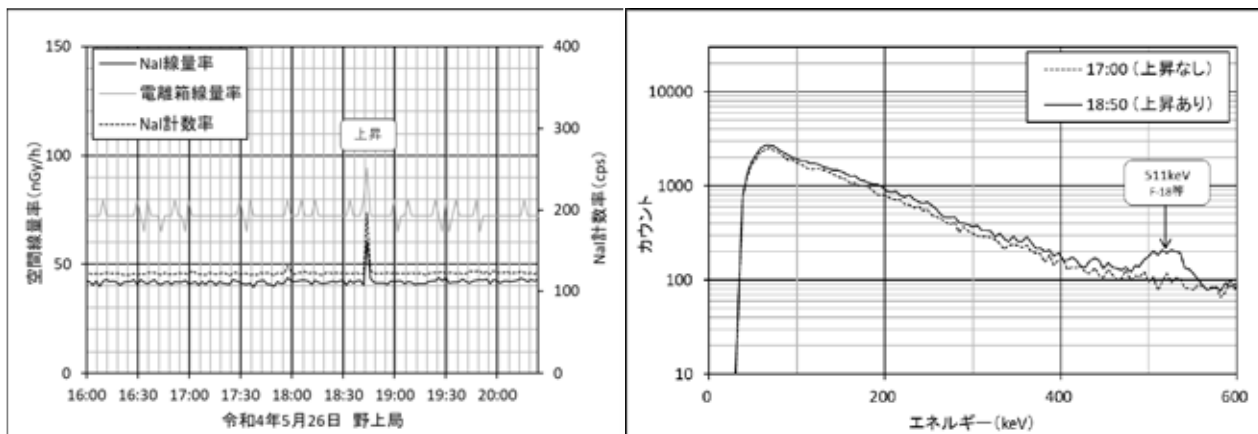
図1 RI (F-18 と推定) 投与者接近による空間線量率 (2分値) の上昇例 左:トレンドグラフ 右:MCA スペクトルグラフ (野上局:令和4年5月26日)
