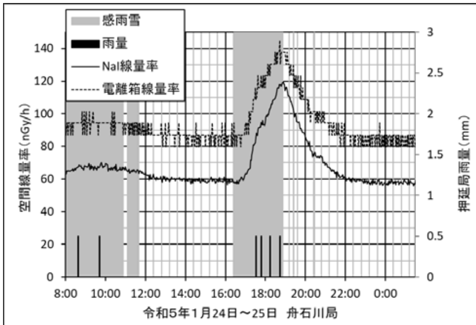
図3 空間線量率（2分値）の上昇
