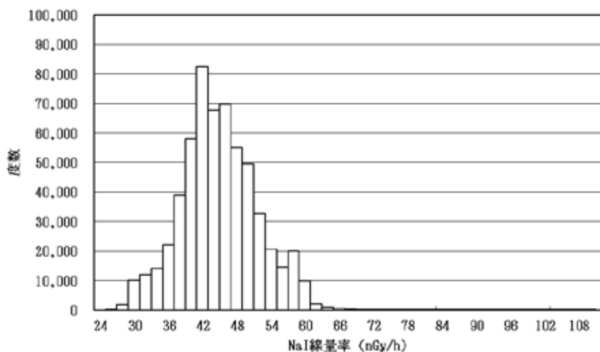
図1 空間線量率度数分布 (NaI 線量率)
