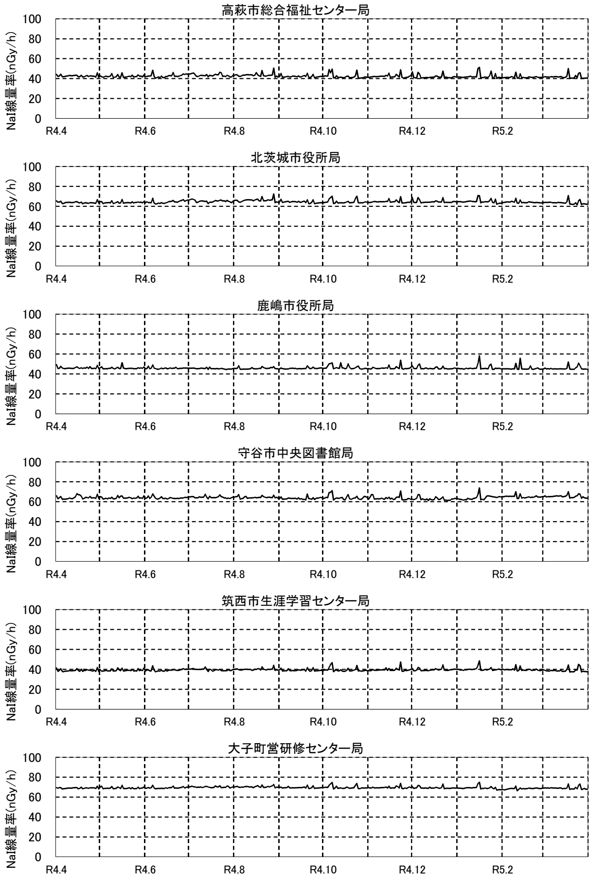
図1 NaI線量率(日平均値)の年間系列変動 (2/2)
