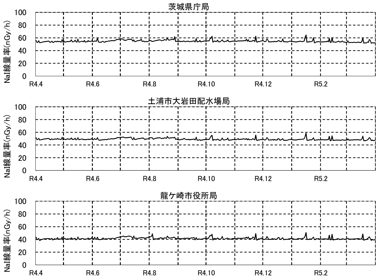
図1 NaI線量率(日平均値)の年間系列変動(1/2)
