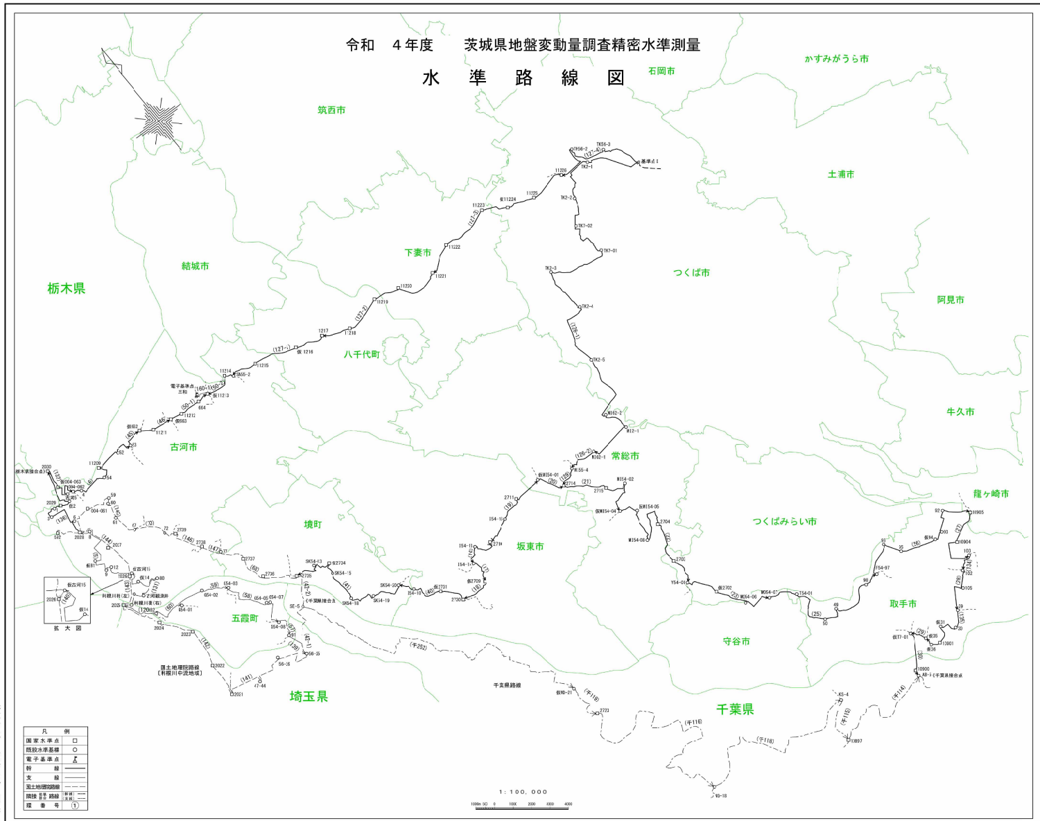
令和4年度 水準路線図
