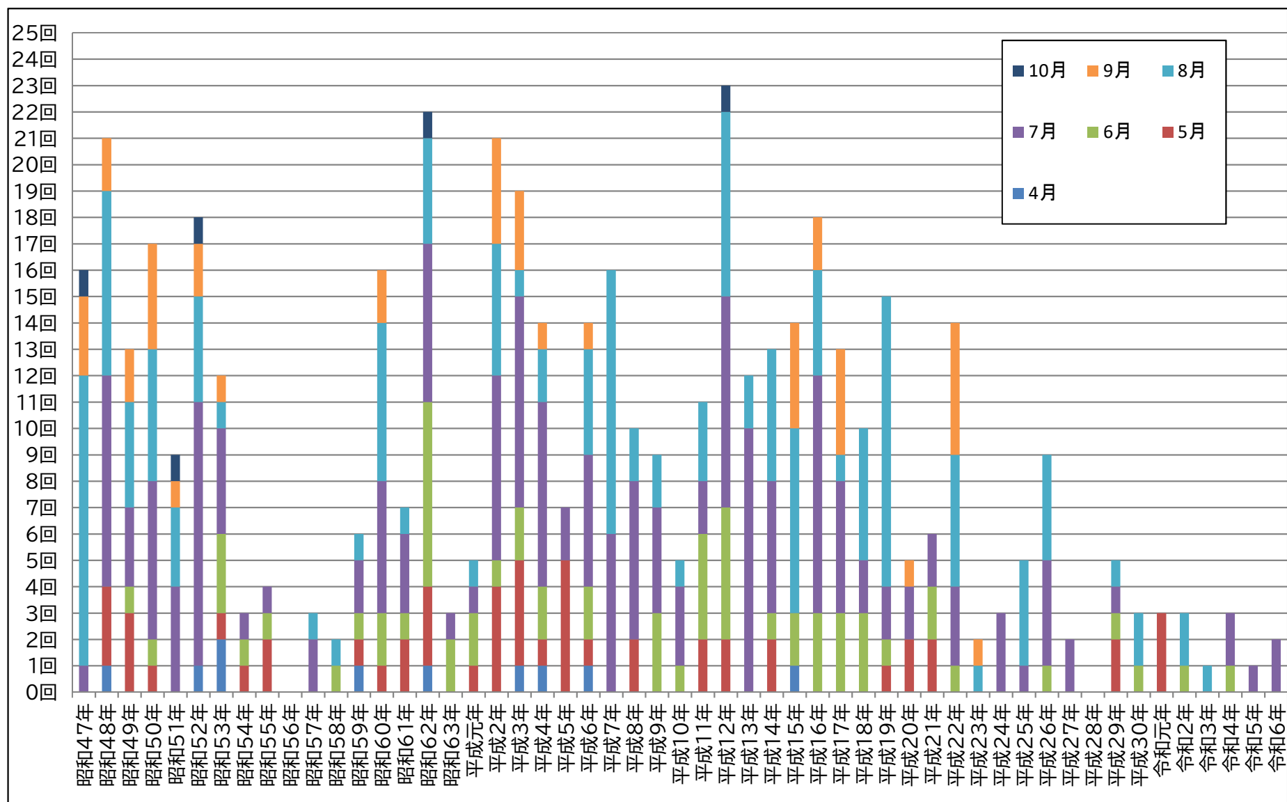
図A 光化学スモッグ注意報の発令日数の推移
