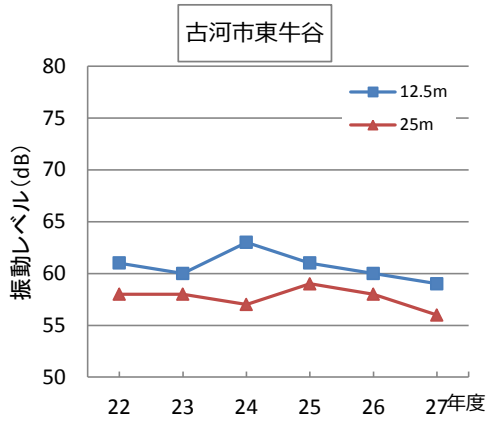
測定地点別振動レベルの経年変化
