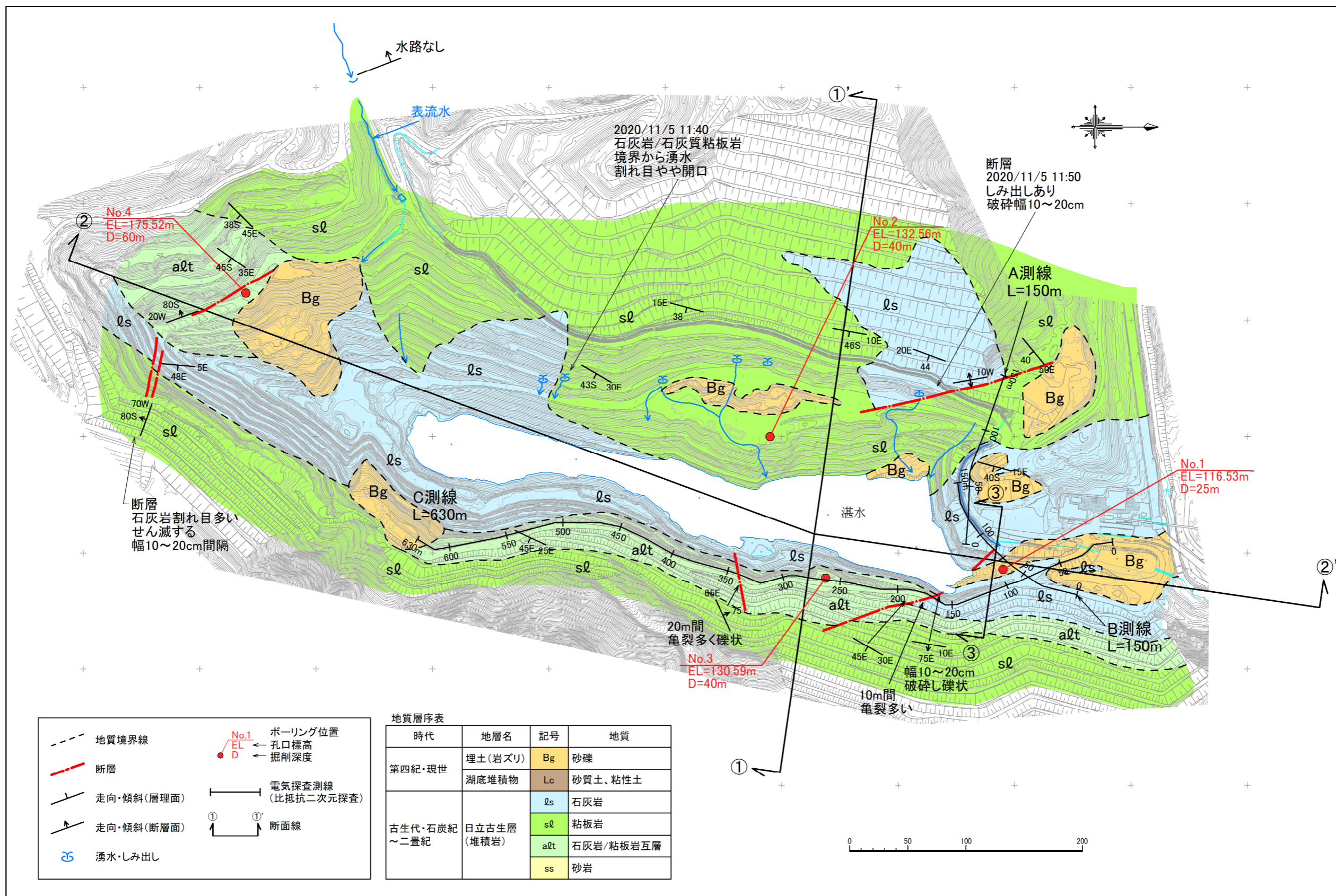
図 1.1.1 ボーリング調査位置図
