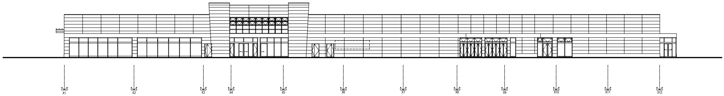
西立面图
