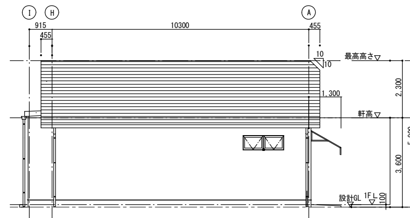
西立面图
