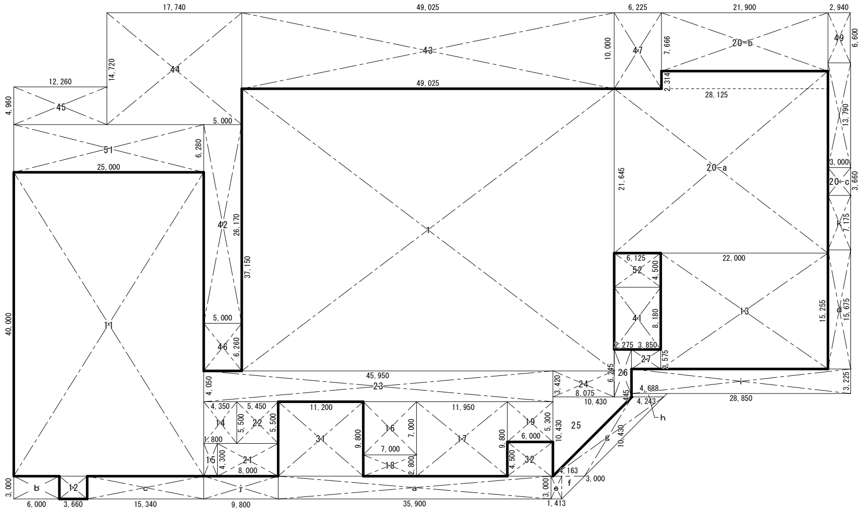
1 階求積図
