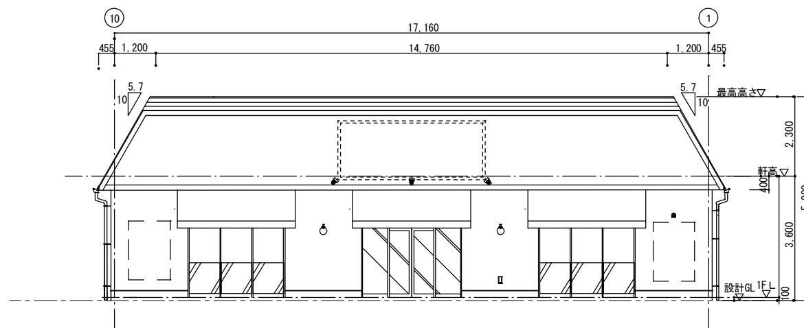
南立面图
