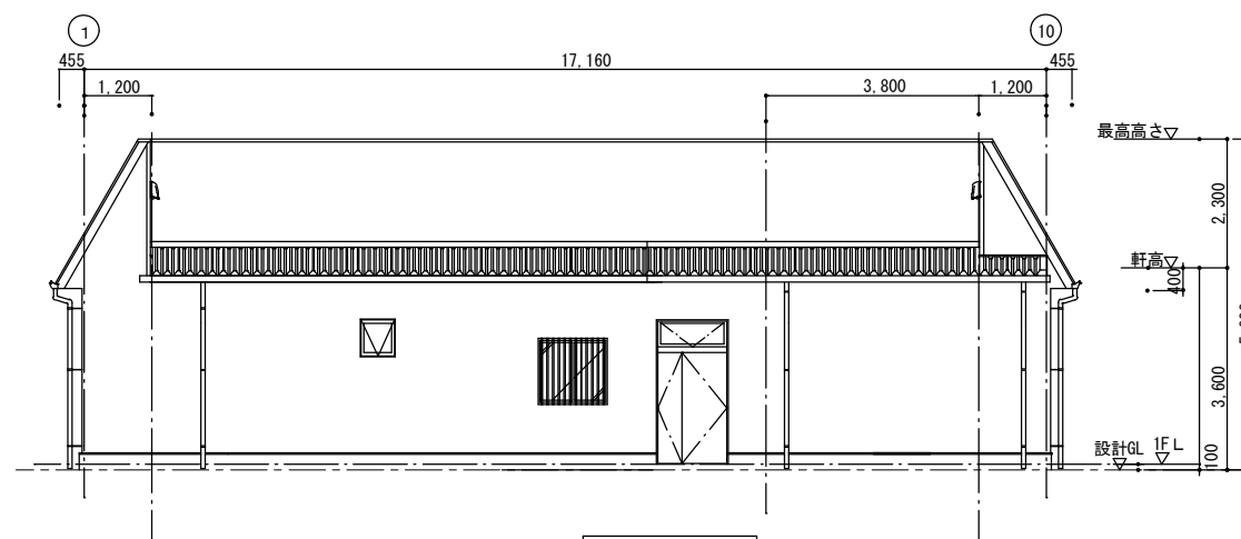
北立面图
