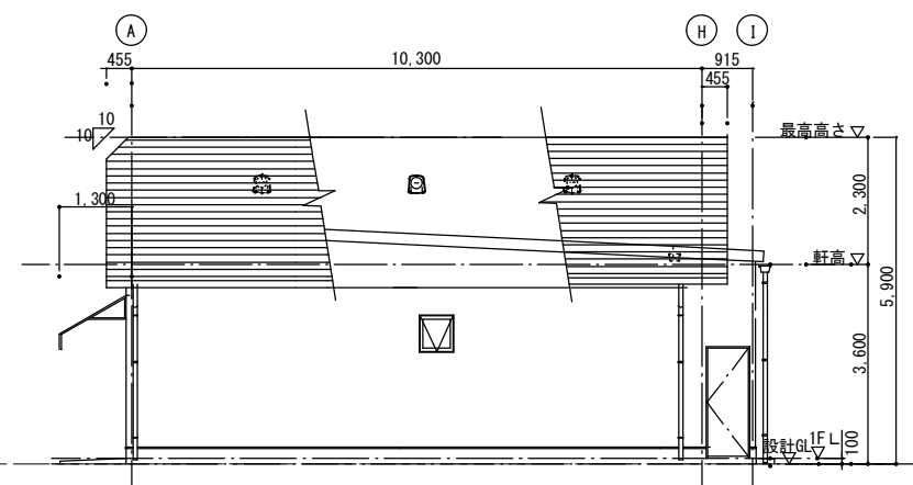
東立面图
