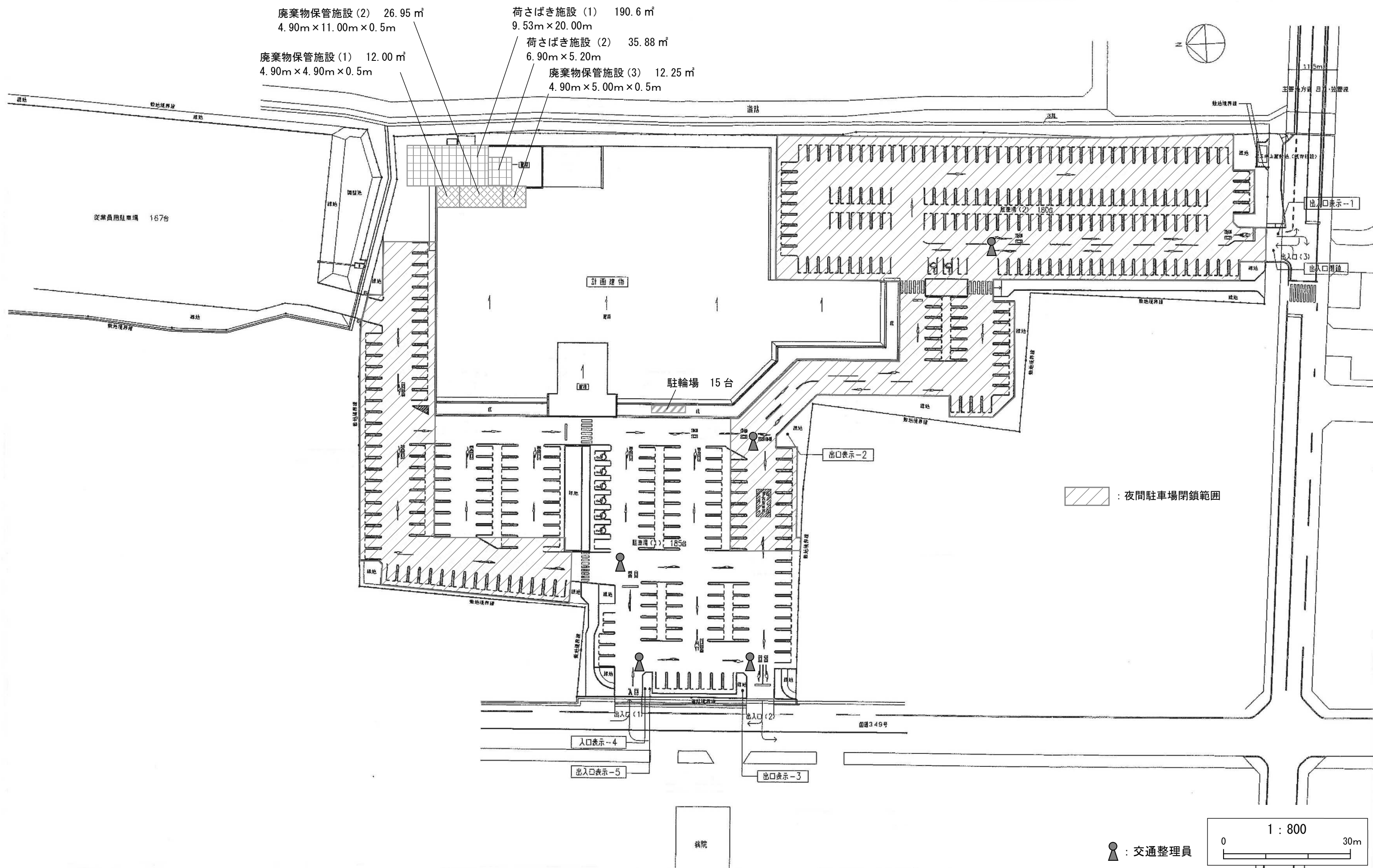
別添図面-3 建物配置図 (変更前)
