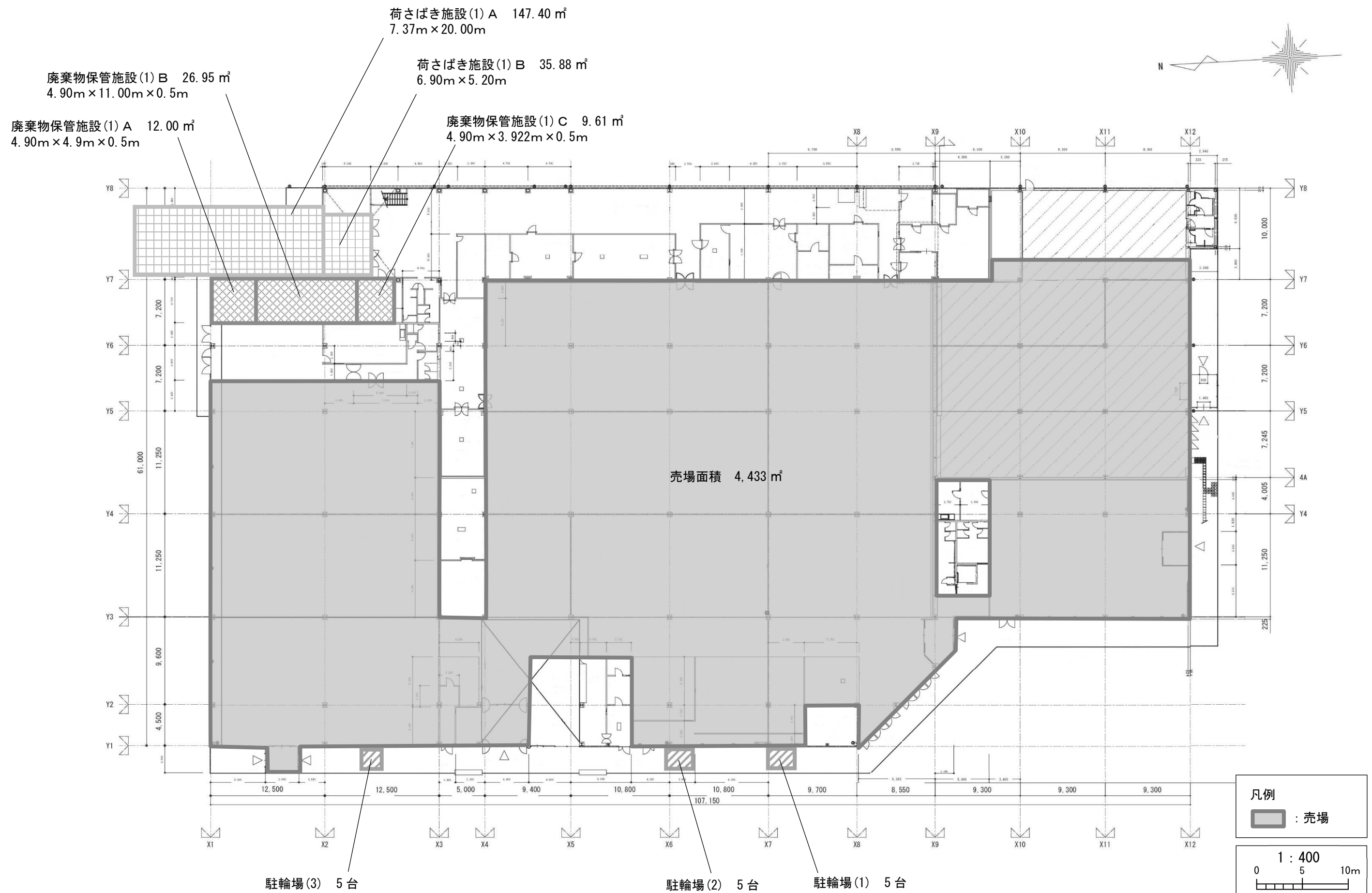
別添図面－6 A棟1階平面図（変更後）
