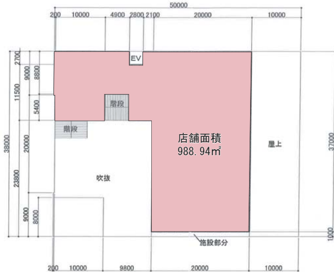
C棟 2階平面図
