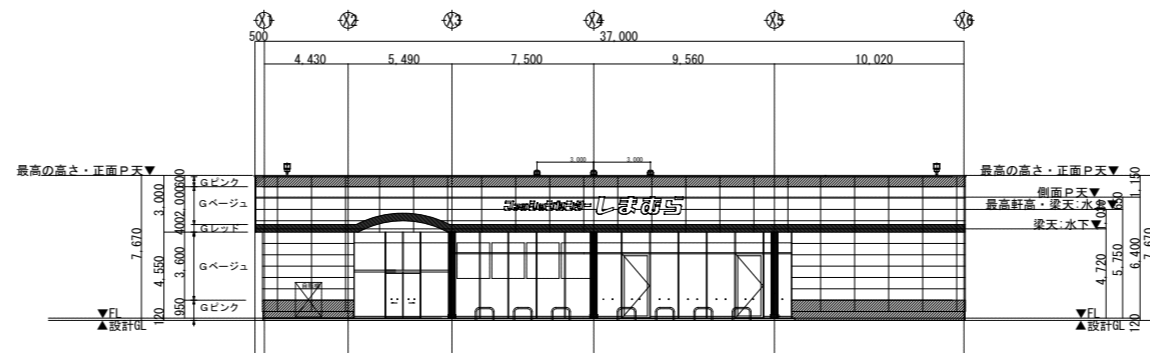
北側立面図
