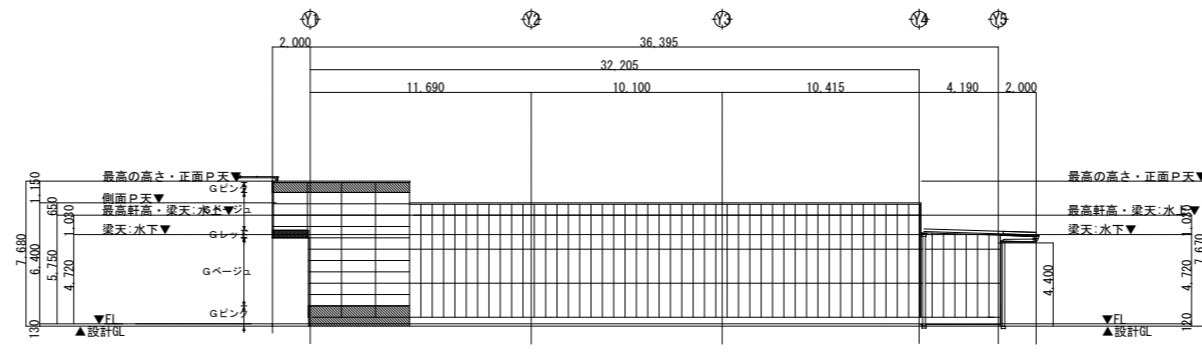
東側立面図
