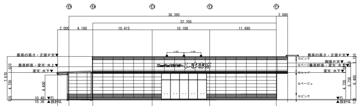
西側立面図
