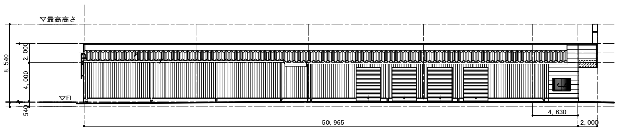
北側立面図
