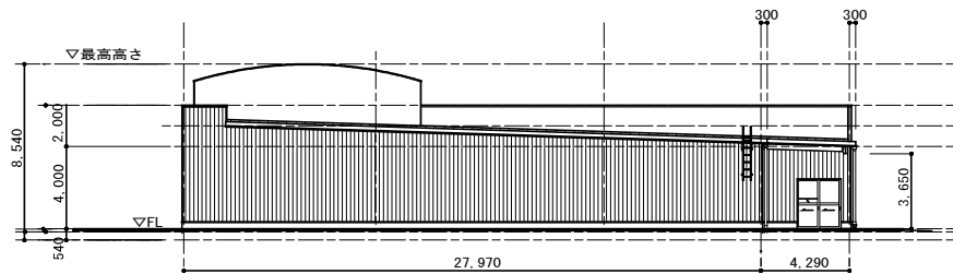
南側立面図
