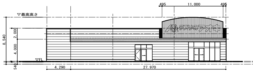
西側立面図
