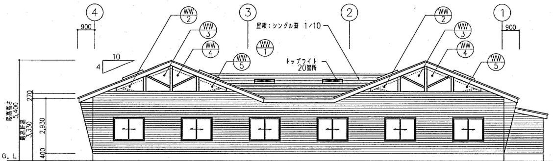
西立面図
