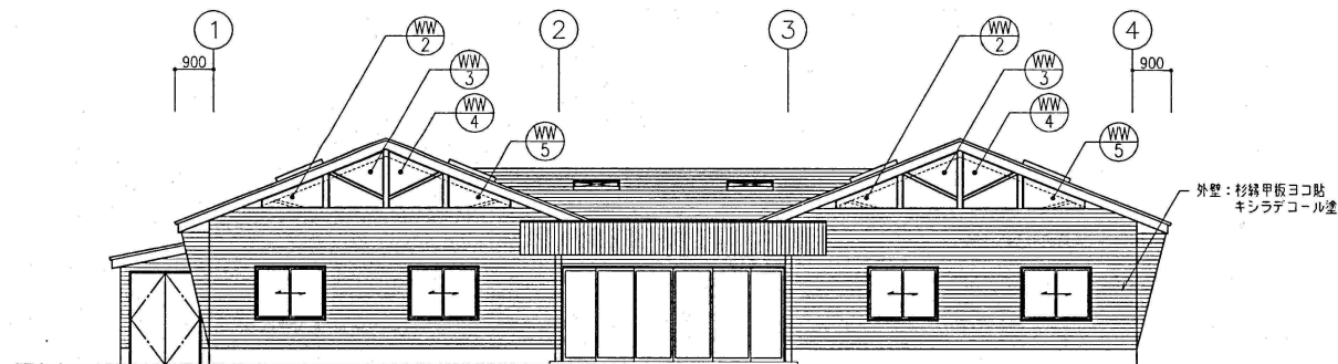
東立面図
