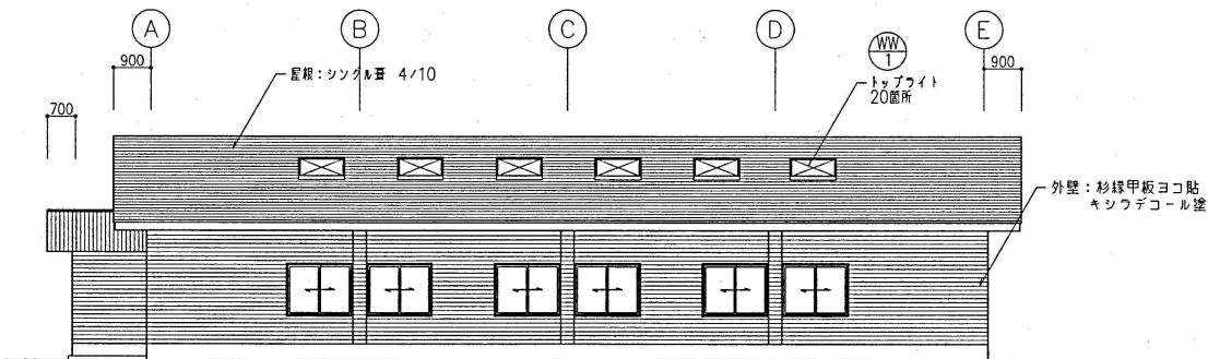
北立面図
