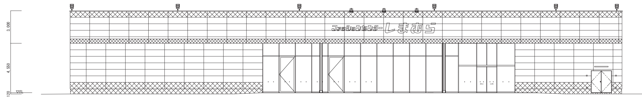
南側立面図
