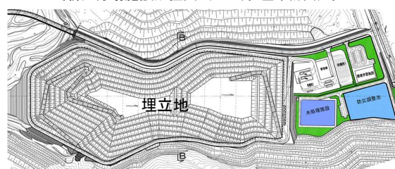
〔新処分場施設配置図 (R4.4月 基本計画)〕
