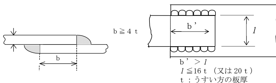
図 11-2-2 前面すみ肉溶接の重ね代 (b) 図 11-2-3 側面すみ肉溶接の重ね代 (b')
