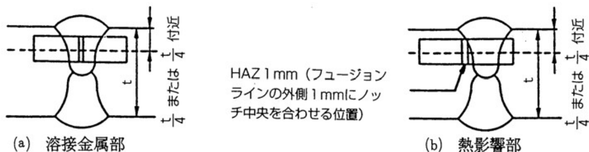
図3-3-2 衝撃試験片採取位置
