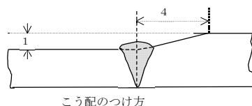
こう配のつけ方 図 11-2-1 勾配のつけ方
