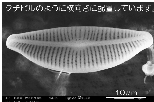
(電子顕微鏡写真) 試料採取 土浦港 2023年8月30日
