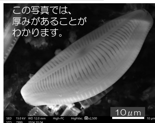
(電子顕微鏡写真) 試料採取 牛久沼 2024年9月18日
