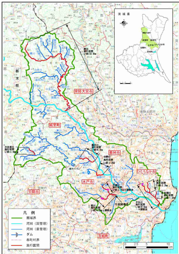
図 2-1 那珂川圏域河川整備の施行区間図
