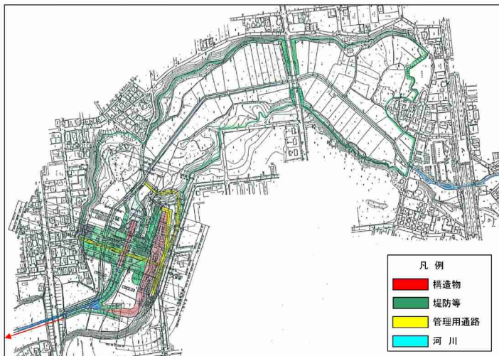
調節池概要図(中丸川)
