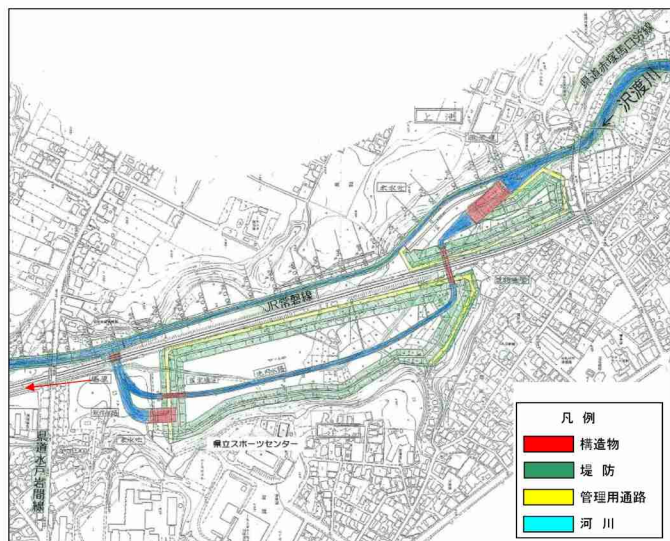
調節池概要図(沢渡川)
